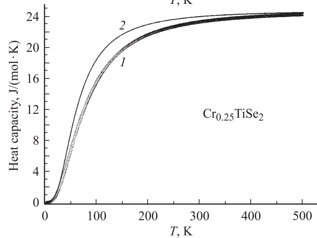
Рис. 2. Типичные температурные зависимости теплоемкости, рассчитанные по плотности фононных состояний. 1 — эксперимент, 2 — аппроксимация в рамках модели Дебая.
